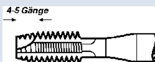
Forma B 4-5 závitů náběh, slamačem třísky
